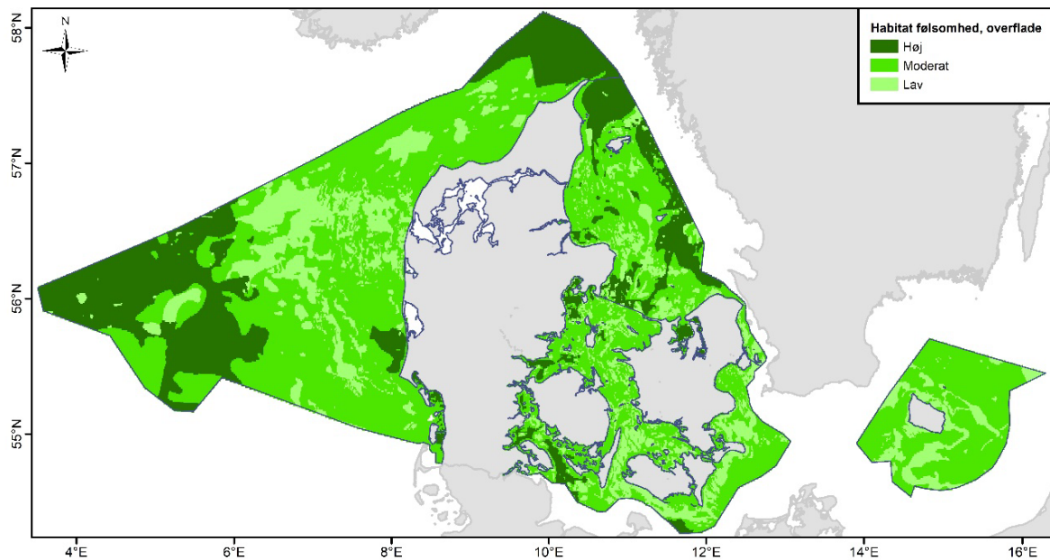
Figur 4.1. Habitatfølsomhed, overflade.
